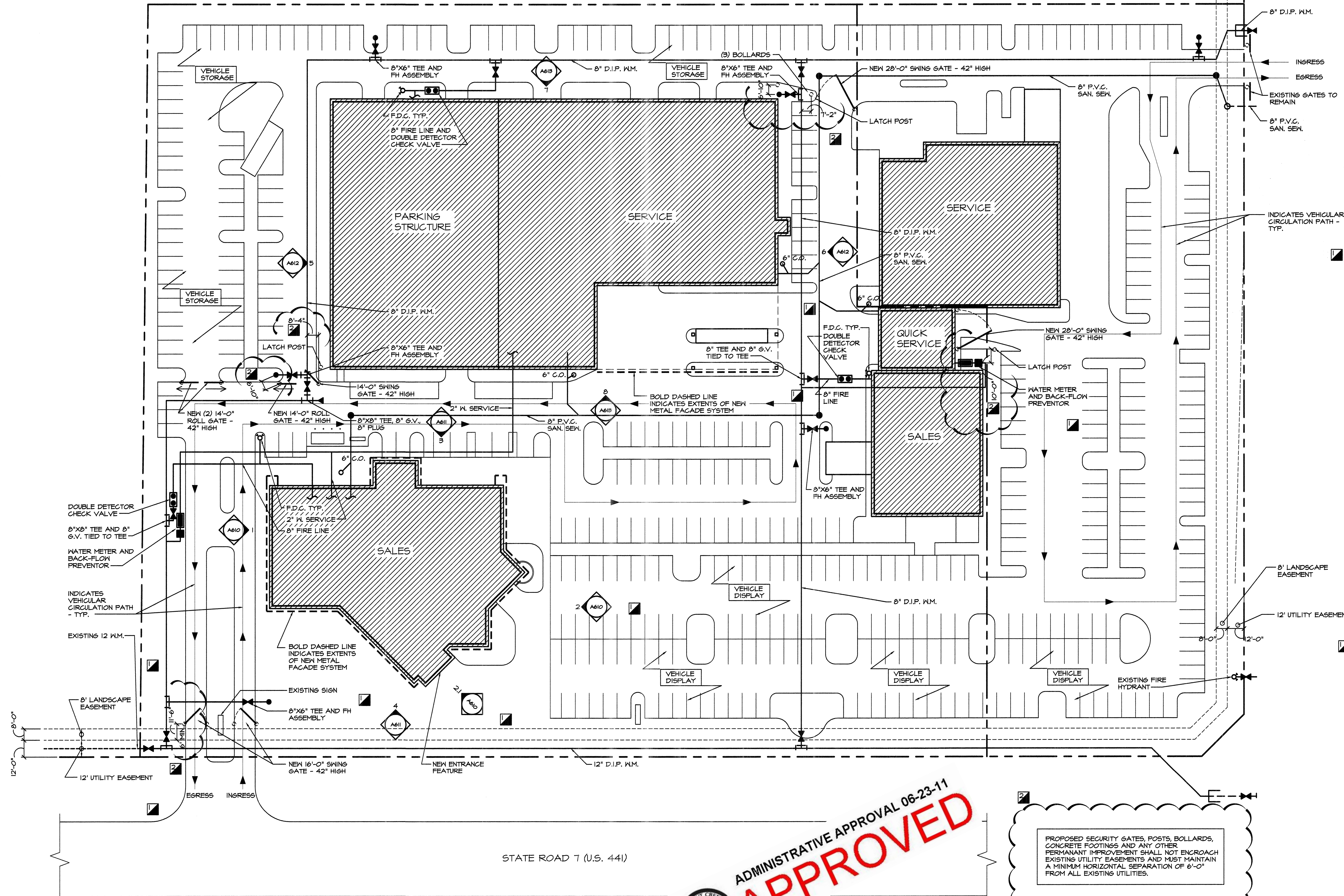
SITE PLAN 1/32"=1'-0"
